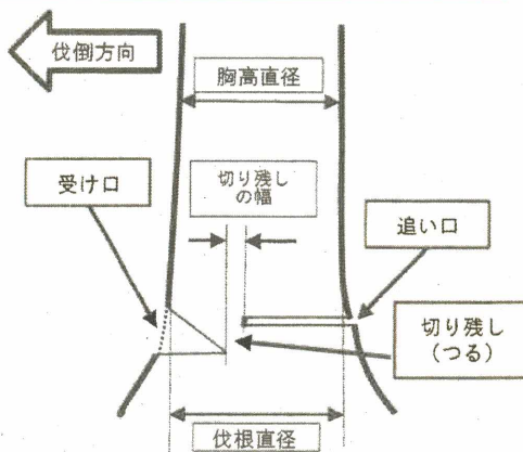
(図1) 受け口、追い口等の関係図
